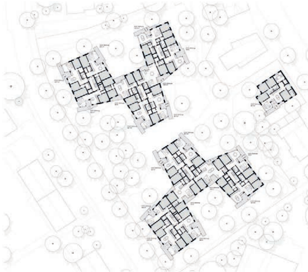
Grundriss Regelgeschoss 1:1000
