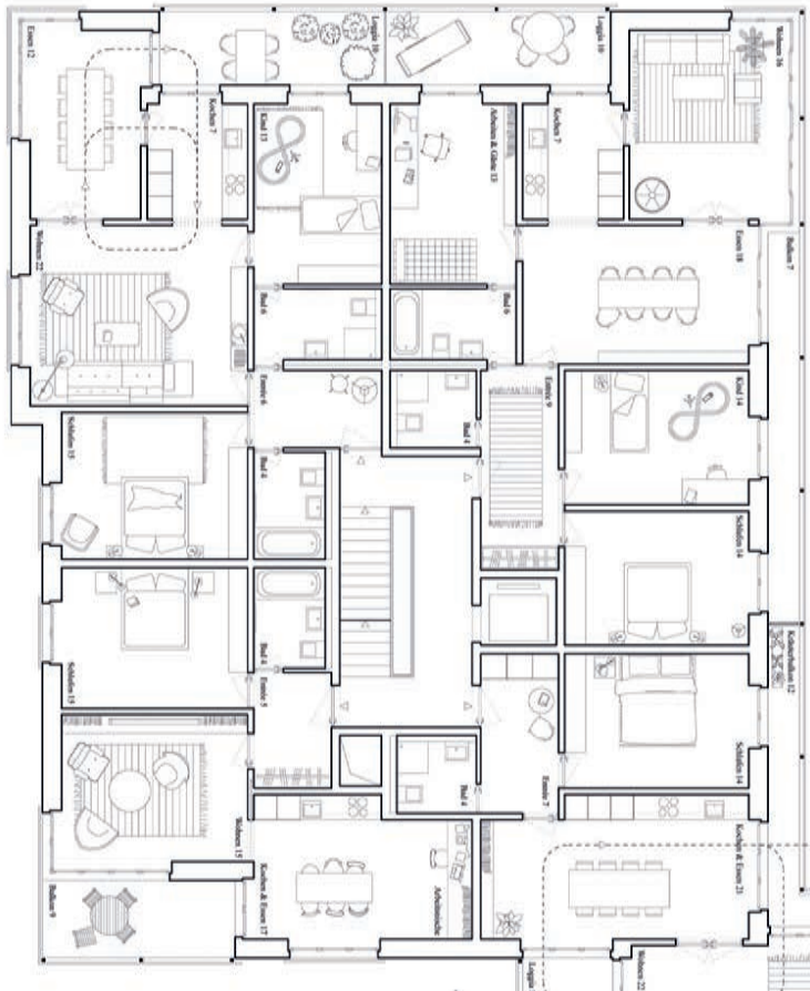
Wohnungstypen 1:200
