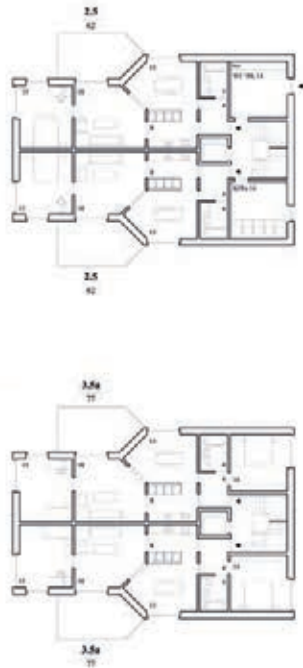
Grundriss Haus Mutschellenstrasse 1:500
