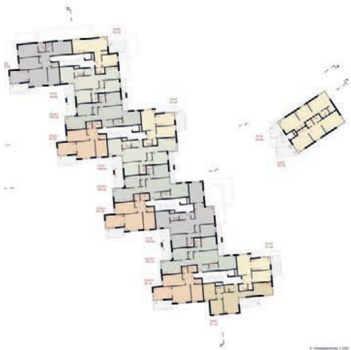
Grundriss 4. Obergeschoss 1:1000
