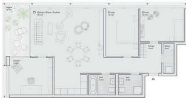
I 4.5-ZIMMERWOHNUNG, TYP A, 101 m²
