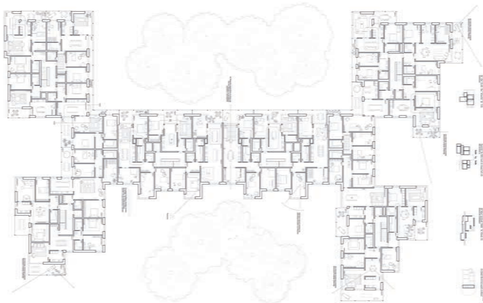
Grundriss Regelgeschoss 1:500
