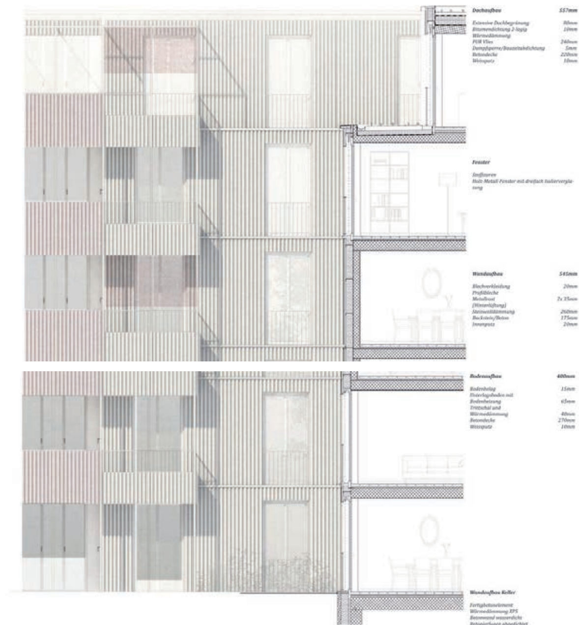
Detailschnitt Fassade 1:100
