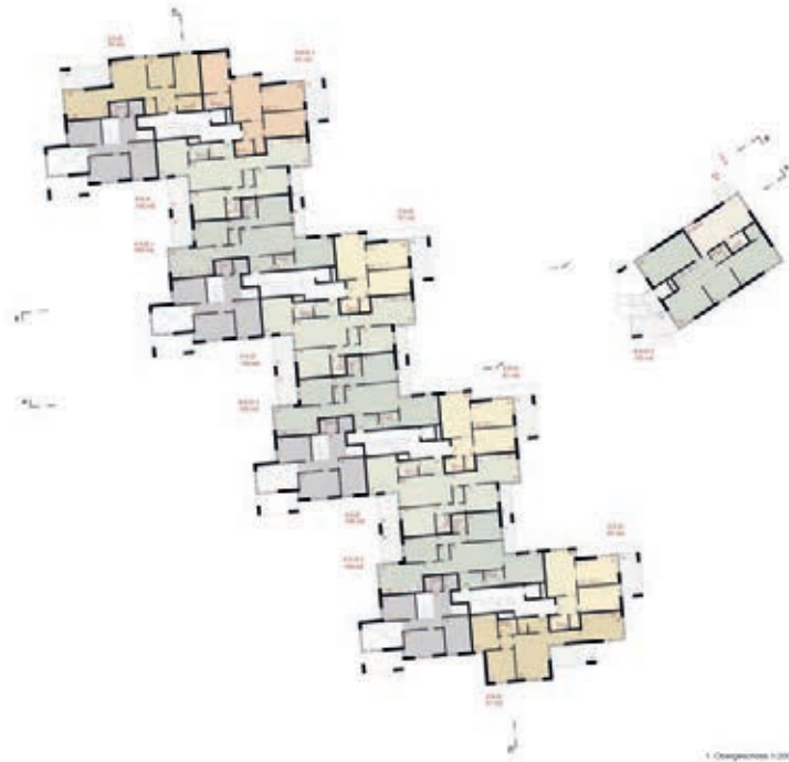
Grundriss 1. Obergeschoss 1:1000
