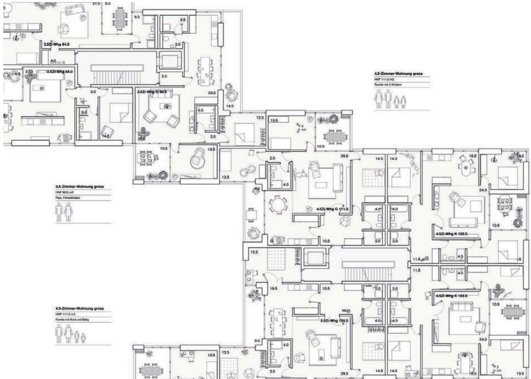
Wohnungstypen 1:200
