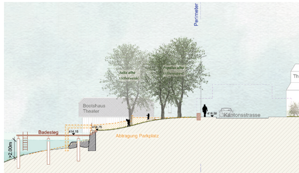
Schnitt C-C', Naberi 1:500
