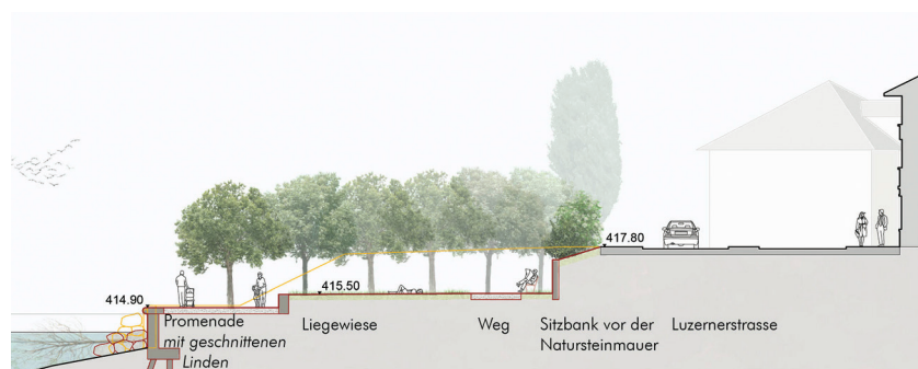
Schnitt C-C', Naberi 1:500
